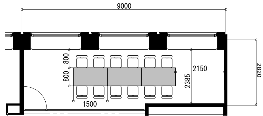
Room G 12名席
